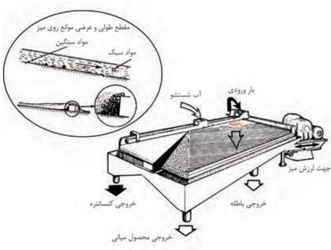
شکل ۱۲- قسمت‌های مختلف میز لرزان
