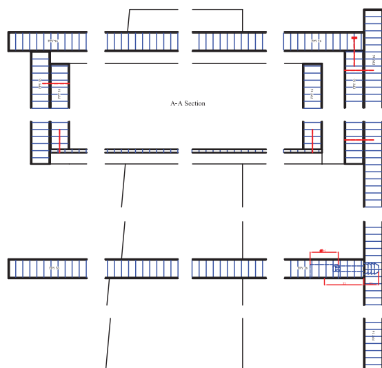
شکل ۸-۵ برش عمودی
