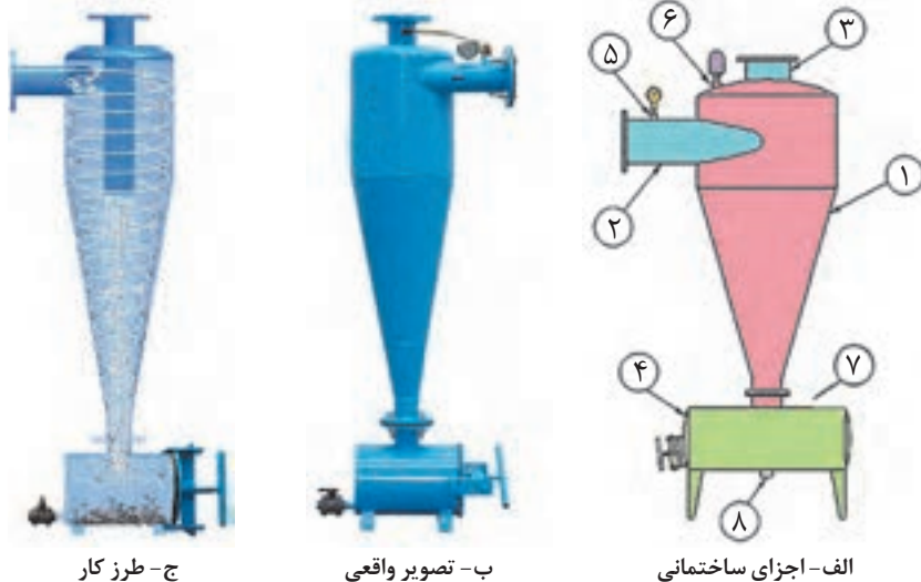
شکل ۵۲-۵. هیدروسیکلون
