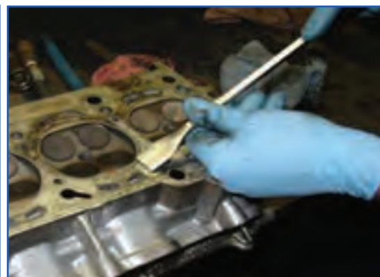
شکل ۴۲-۴ واشر سرسیلندر چسبیده به سیلندر
