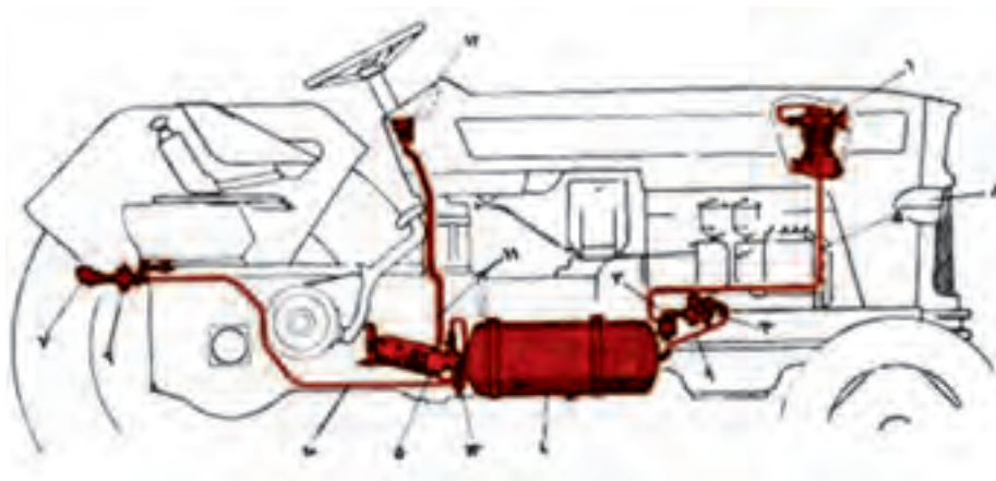
شکل ۱-۸ - اجزای مدار کمپرسور باد
