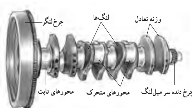
شکل ۲-۳۴- اجزای میل لنگ
