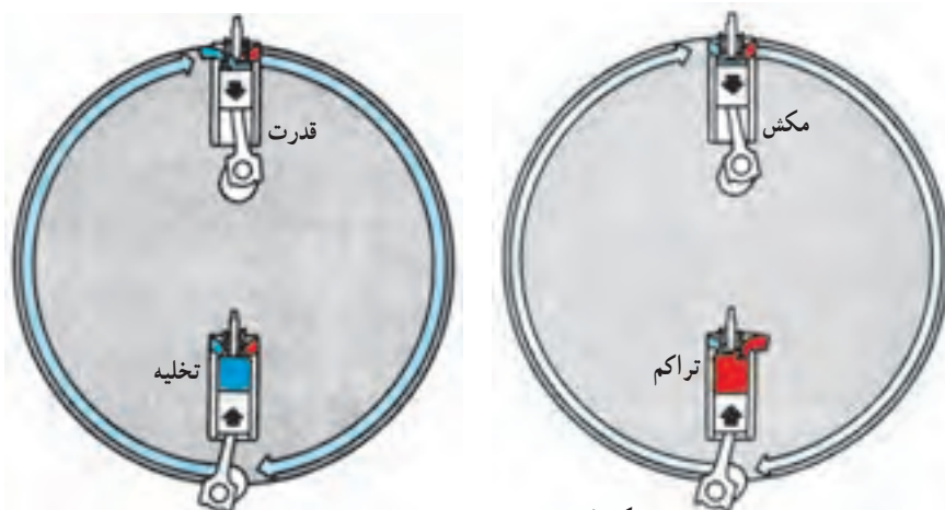
شکل ۶-۱- چرخه موتور چهار زمانه
