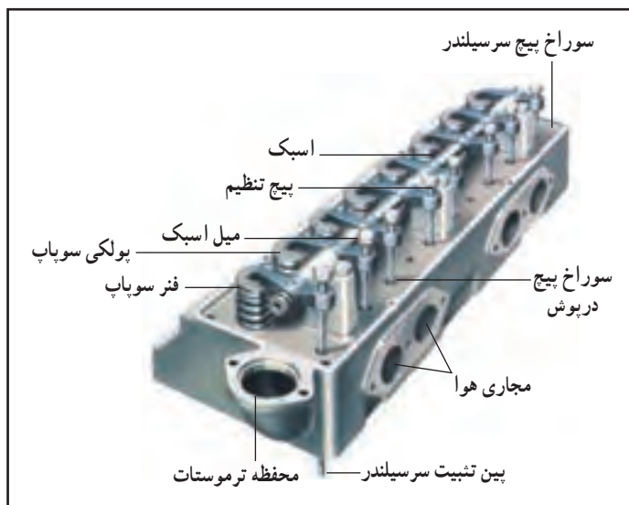
شکل ۴-۲- اجزای سرسیلندر
