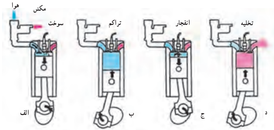
شکل ۷-۱ - چهار زمان کار موتور چهار زمانه بنزینی
