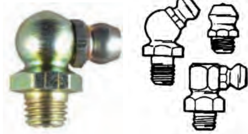
شکل ۵۴-۷- انواع گریس خور از نظر زاویه قرار گرفته
