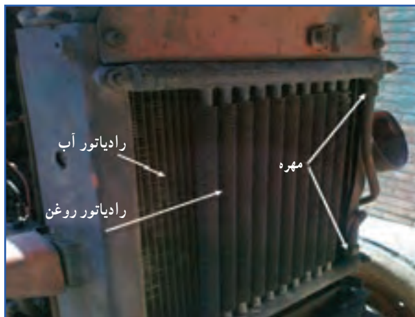
شکل ۳۶-۷- رادیاتور روغن
