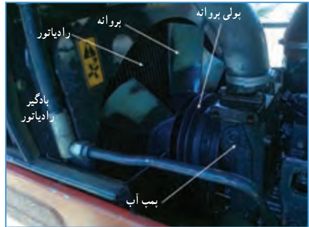
شکل ۳۴-۲- رادیاتور تراکتور MF285
