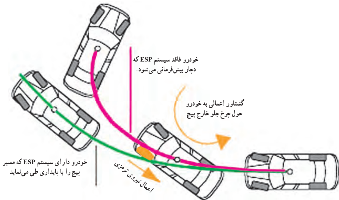
شکل ۱۹-۱۱- عملکرد سیستم کنترل پایداری در حالت بیش فرمانی خودرو
