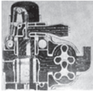
شکل ۱-۱۸- مرحله‌ی تخلیه و شستشوی سیلندر دیزل دوزمانه‌ی GM
