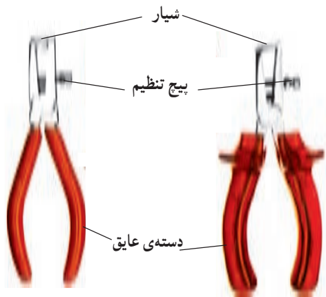
الف — سیم لخت‌کن دسته عایق قوی ب — سیم لخت‌کن دسته عایق فشار معمولی شکل ۱-۶ — دو نمونه سیم لخت‌کن ساده
