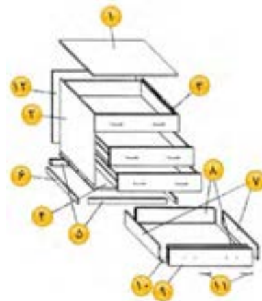
شکل ۲-۱۲- پرسپکتیو انفجاری از یک دراور.
