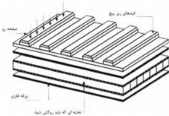
شکل ۳-۶- با قرار دادن صفحات کمکی مکم بر رو و زیر صفحه‌ی مورد نظر، عمل پرس‌کاری انجام می‌شود.
