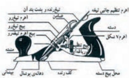
شکل ۲-۳- رنده‌ی دو تیغ فلزی
