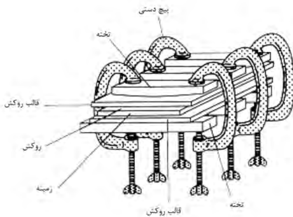
شکل ۴-۶- عمل پرس‌کاری، به وسیله‌ی پیچ‌دستی‌های G شکل و صفحات کمکی انجام می‌شود.
