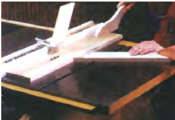
شکل ۱۲-۹۱- برش قطعات MDF با مفاظ و وسایل ایمنی.
