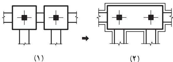
شکل ۱-۵۴ پی مشترک مستطیل
