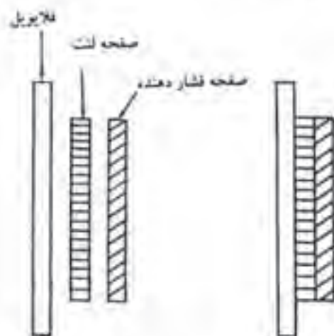
شکل ۷-۴ نحوه عملکرد کلاچ
