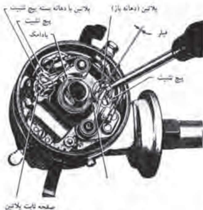
شکل ۳۸: تنظیم دهانه پلاتین
