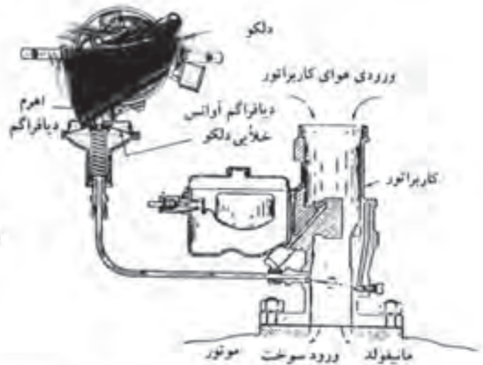
شکل ۴-۱۰: عملکرد دستگاه آوانس خلائی (شکل از کمپانی فورد)
