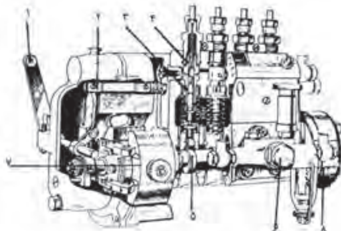
۱- اهرم تنظیم ۲- میل دنده گاز ۳- واحد پمپ ۴- سوپاپ فشار ۵- میل بادامک ۶- پمپ سوخت رسان ۷- رگولاتور حرارت از مرکز ۸- تنظیم کننده سوخت پاشی
