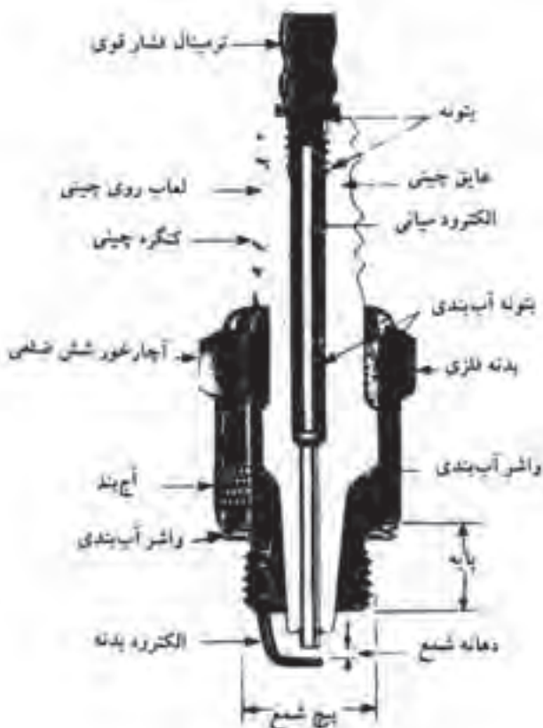
شکل ۴-۱۲- ساختمان شمع
