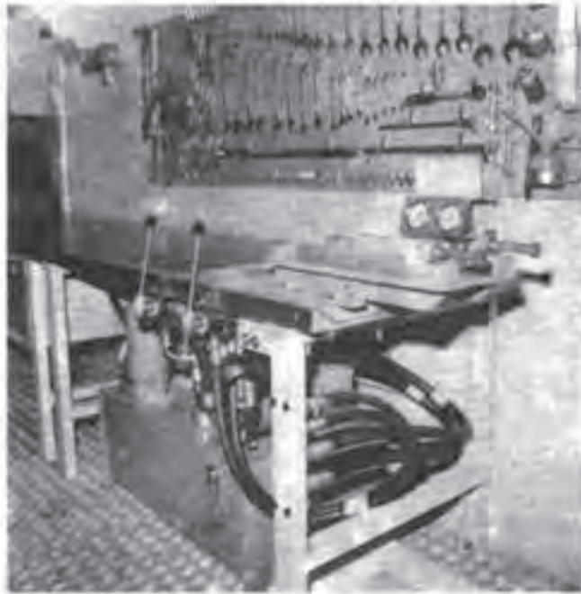
شکل ۱۸-۲: نمای میز کار و تابلو ابزار یک تعمیرگاه سپار ویژه تعمیر ماشینهای معدنی در نقاط دور افتاده
