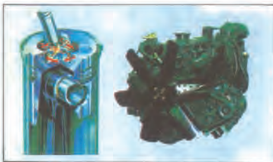
شکل ۲-۱: نمای خارجی موتور نصب شده روی ماشین اکسکواتوری که در شکل ۲-۲ در حین کار مشاهده می‌شود. (سیلندر و پیستون آن در قسمت چپ تصویر آمده است.)
