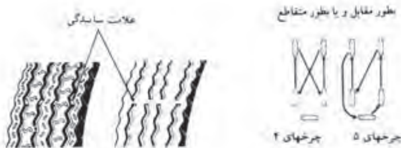
شکل ۱۰-۴: نحوه تمویض جای لاستیکها و تشخیص ساییدگی آنها
