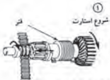
حرکت پنیون به سمت دنده فلاپویل جهت درگیری - در شروع استارت -
