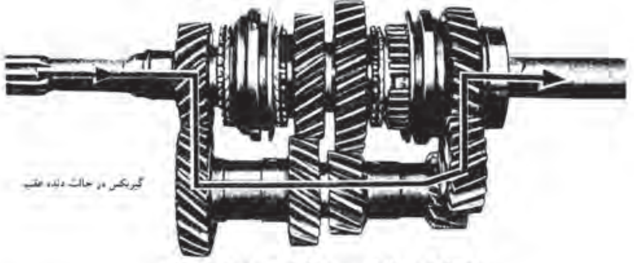
دنباله شکل ۱۵.۷ نحوه درگیری دنده‌های گیربکس ۳ دنده‌ای (موتور شورولت)
