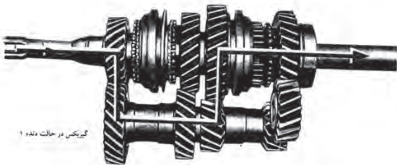
شکل ۷۰۵. نحوه درگیری دنده‌ها
