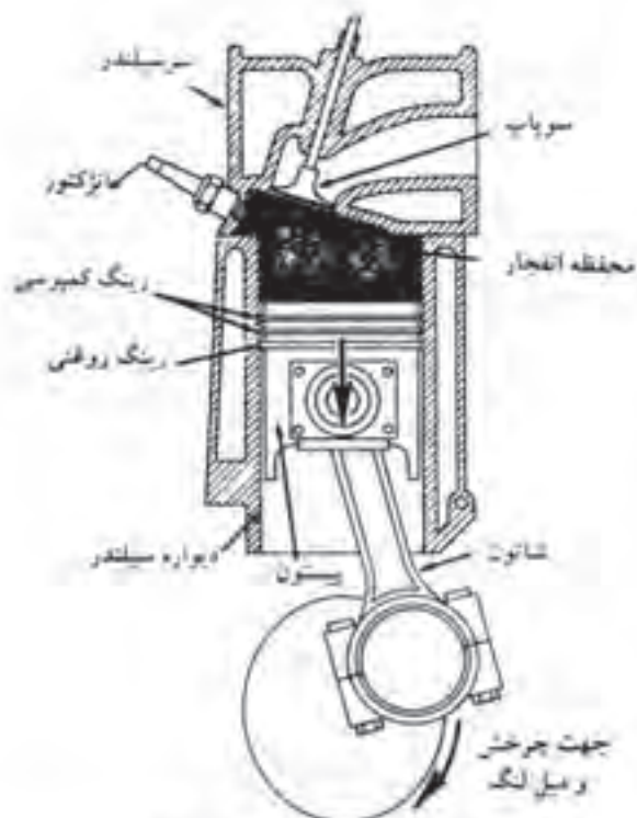
شکل ۹-۳ یک سیلندر از موتور دیزلی
