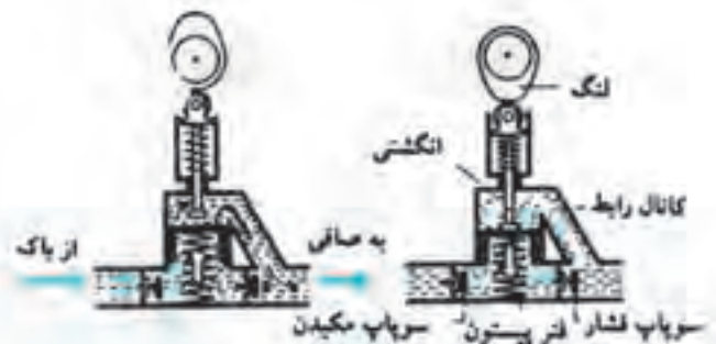
شکل ۹-۴ پمپ سوخت رسانی
