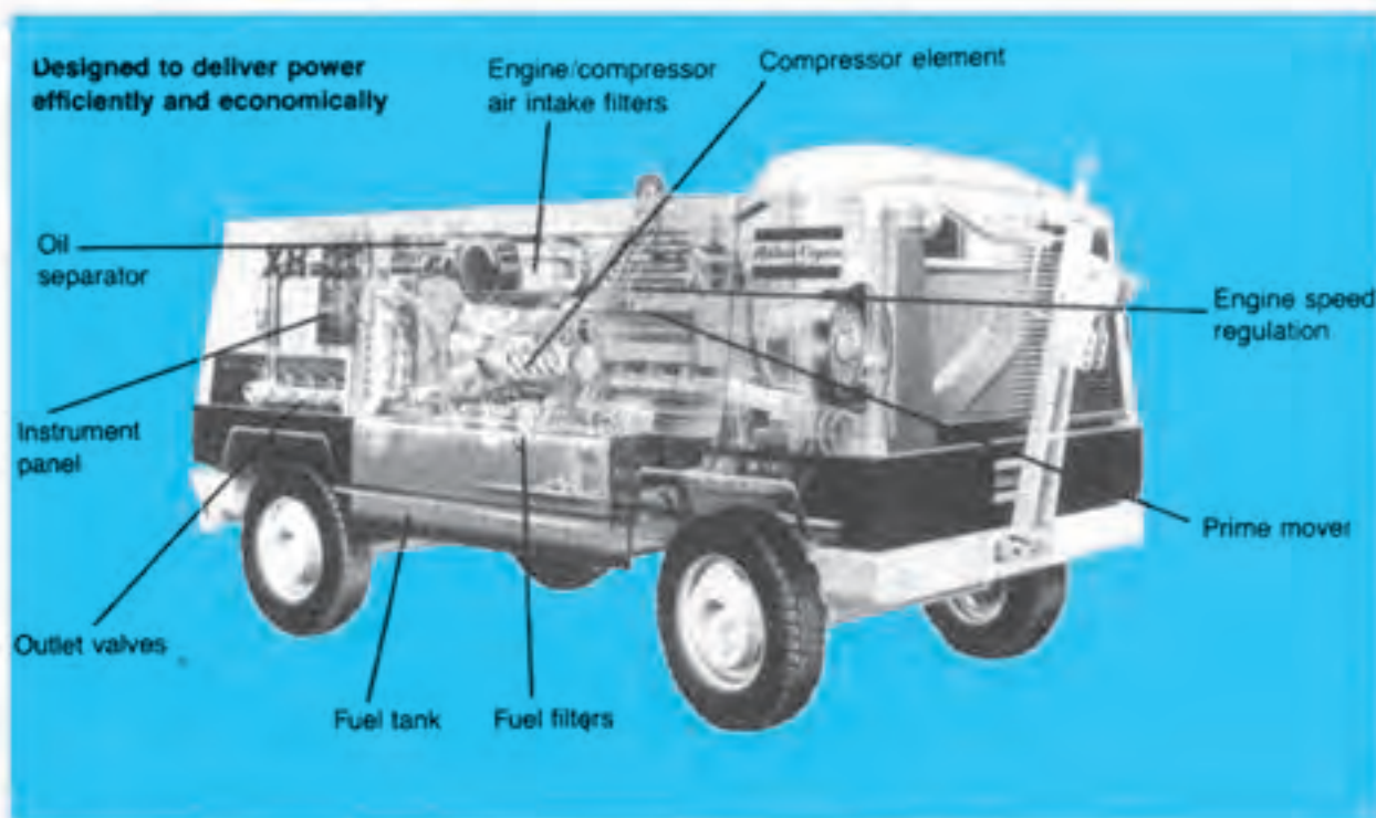
قسمتهای مختلف کمپرسور متحرک «اگلنس کوپکو» با موتور دیزلی
