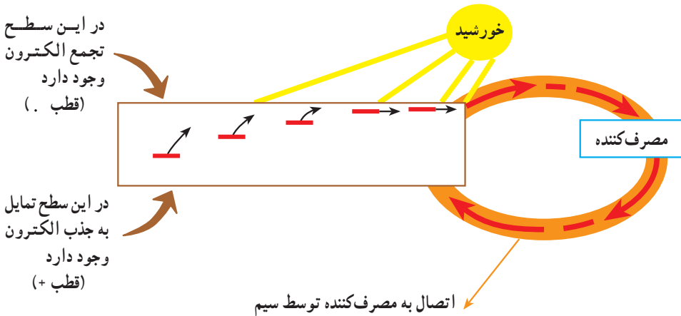
شکل ۸-۳ طرز کار یک سلول فتوولتائیک
