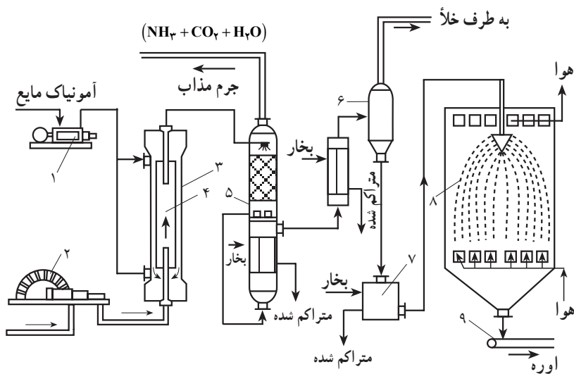
شکل ۴-۵ فرآیند تهیه اوره
