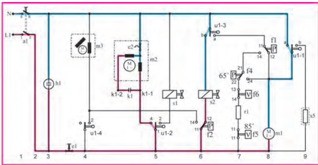
ت - نقشه تفکیکی مدار الکتریکی ماشین ظرفشویی اتوماتیک با الکتریمپ دو جهته در مقطع زمانی ۱۲
