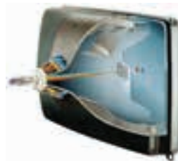
شکل ۴-۹ تصویر یک لامپ اشعه‌ی کاتدی
