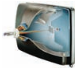
شکل ۹-۴ تصویر یک لامپ اشعه‌ی کاتی
