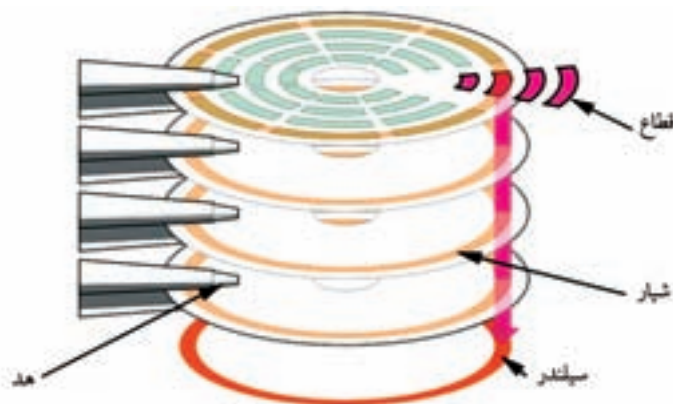
شکل ۱۰-۳ سیلندر
