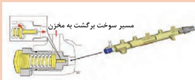
شکل ۱۵- سوپاپ کنترل فشارمکانیکی در تزریق ریل مشترک
