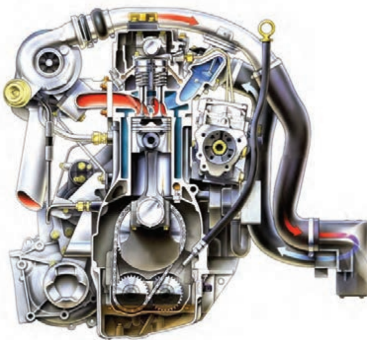
شکل ۱- مقطع عرضی برش خورده یک نوع موتور دیزل
