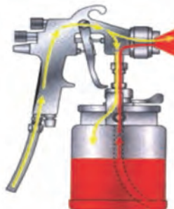
شکل ۱۶۵- پیستوله کاسه بالا
