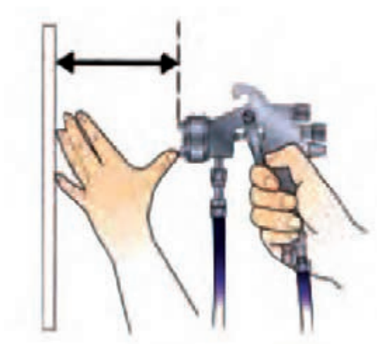
شکل ۴۵- الف) رعایت فاصله پیستوله با سطح کار
