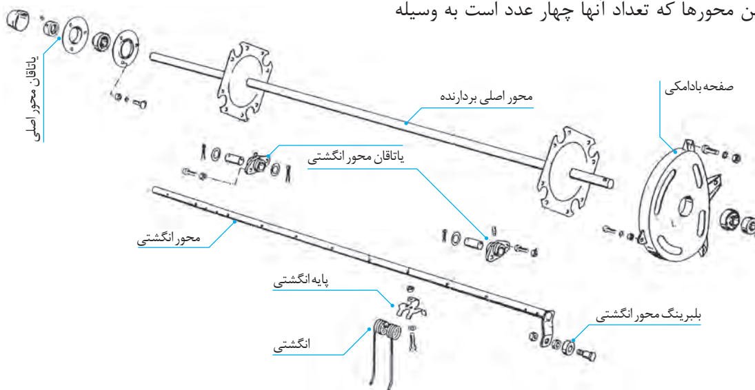
شکل ۲- قطعات متحرک بردارنده
