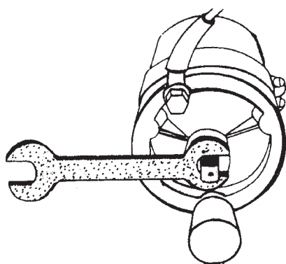
شکل ۴۵- آزاد کردن دنده استارتر
