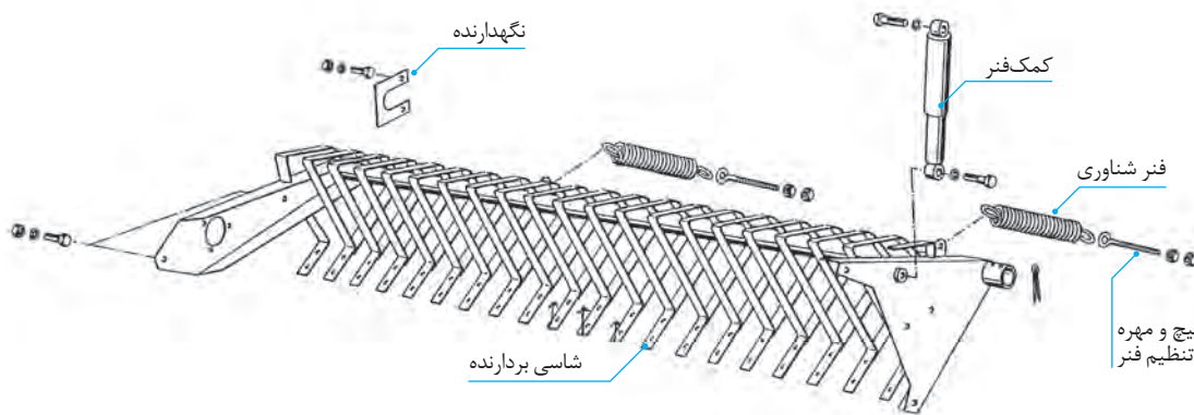
شکل ۱- شاسی بردارنده و متعلقات آن
