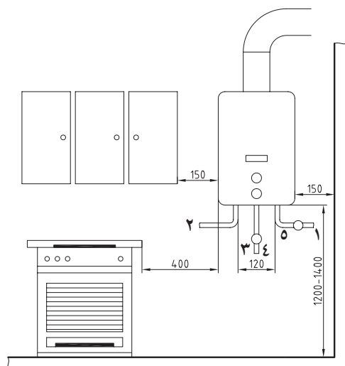
شکل ۱-۸ نقشه نصب آب گرم کن گازی دیواری.
