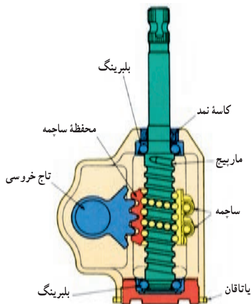
شکل ۲-۱۱- جعبه فرمان ساچمه‌ای
