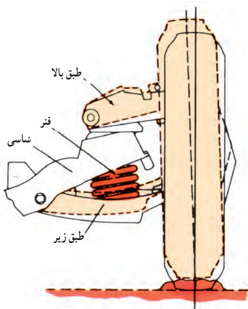
شکل ۲۰-۳ نوسان زیاد چرخ در سیستم تعلیق مستقل
