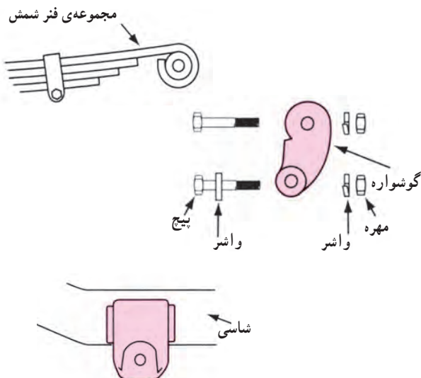
شکل ۳-۱۶ اتصال عقب فنر شمش
