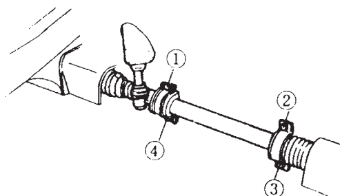
شکل ۲-۵۵- ترتیب بستن پیچ‌ها و بست‌های جعبه فرمان
