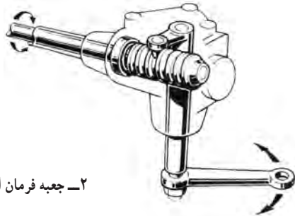
۱- جعبه فرمان حلزونی
