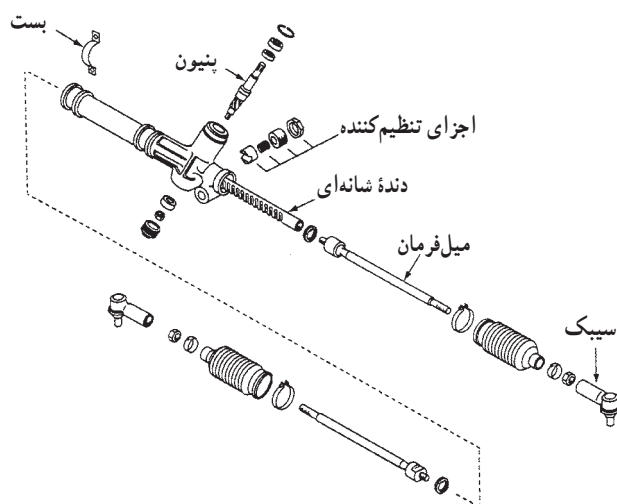
شکل ۲-۹- جعبه فرمان شانه‌ای (کشویی)
