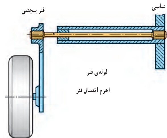
شکل ۲۸-۳ فنر پیچشی
