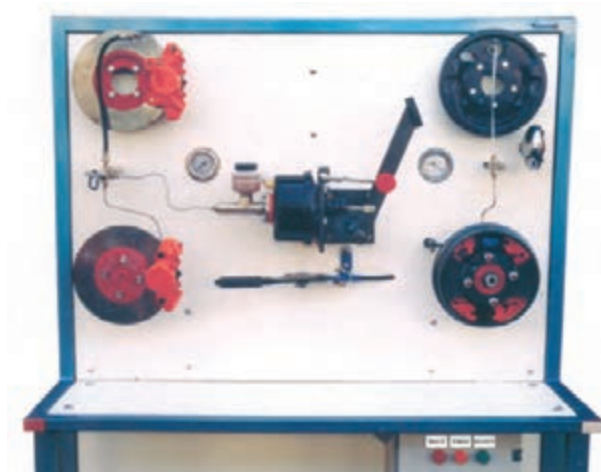
شکل ۱۴-۱- اجزای سیستم ترمز
