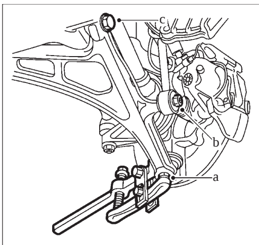
شکل ۱۲۱-۳ جدا کردن سیبک از طبق
