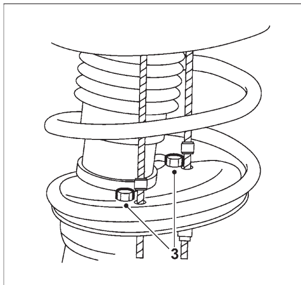
شکل ۳-۱-۴ نصب کابل‌های نگه‌دارنده فنر
