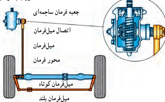
محور جعبه فرمان
