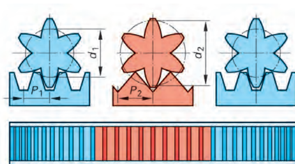
شکل ۲-۱۰- انواع پنیون و دنده شانه‌ای
