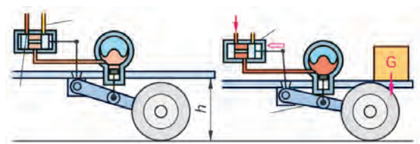
شکل ۳-۳۱- سیستم تعلیق هیدرونیوماتیکی
