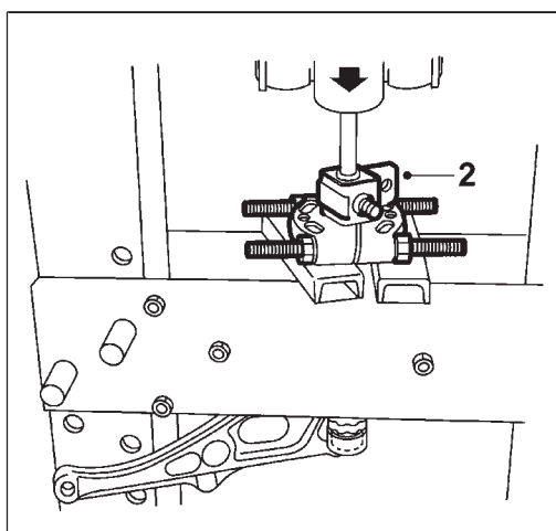
شکل ۱۲۳-۳ خارج کردن بوش لاستیکی عقب
