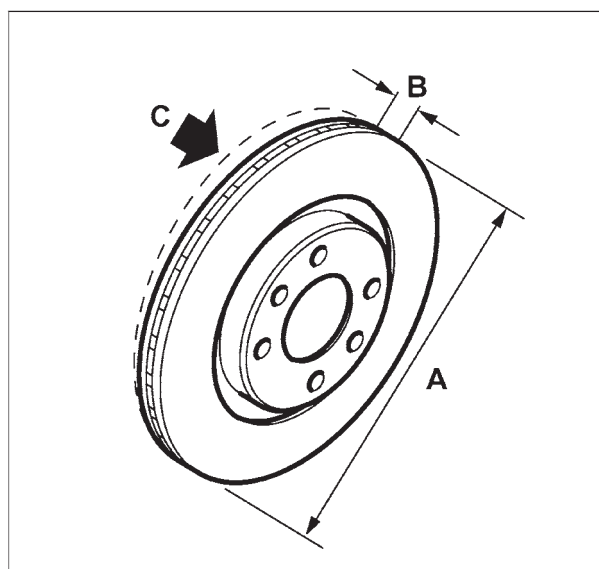
شکل ۱۲۵-۱ اندازه‌های دیسک ترمز
