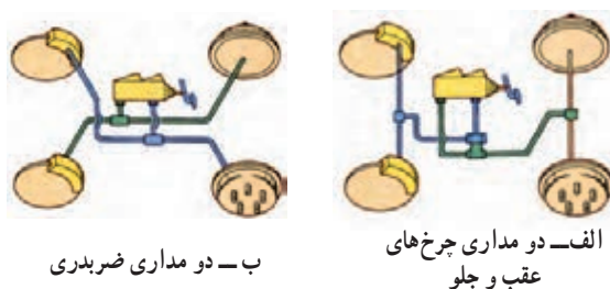
شکل ۱-۲۲ سیستم ترمز دابل (دو مداری)
