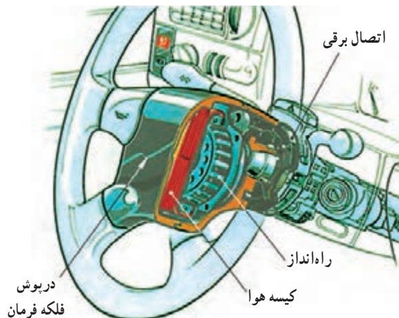
شکل ۲-۲۱- فلکه فرمان با کیسه هوا (Air bag)
