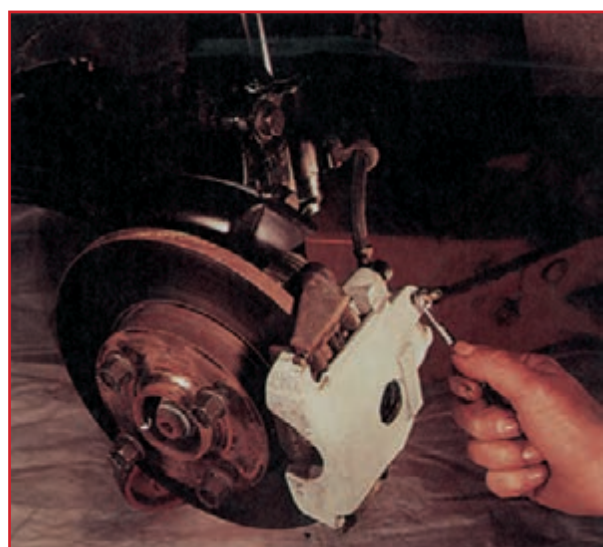
شکل ۱-۶۷- پیچ هواگیری سیلندر چرخ
