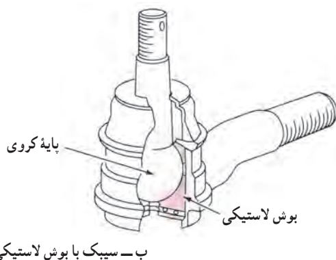
شکل ۲۸-۲- انواع سیبک
