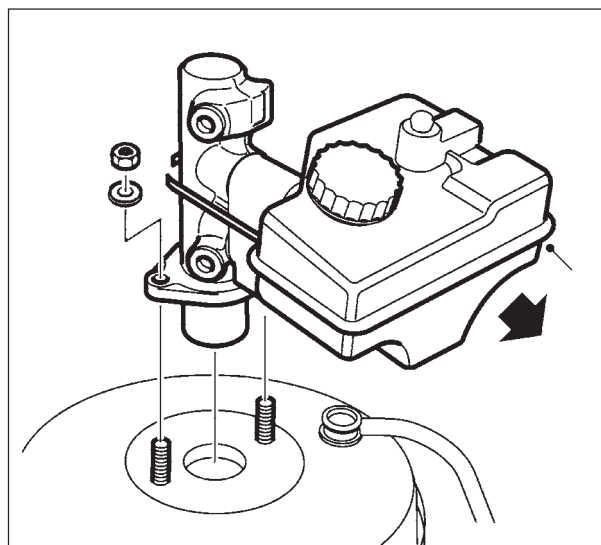
شکل ۱-۱۲۹- جدا کردن سیلندر اصلی از بوستر
