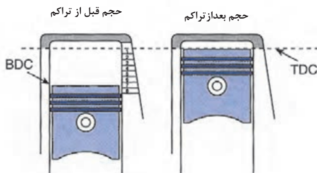
نسبت تراکم
