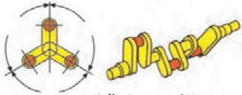
میل لنگ موتور شش سیلندر V شکل
