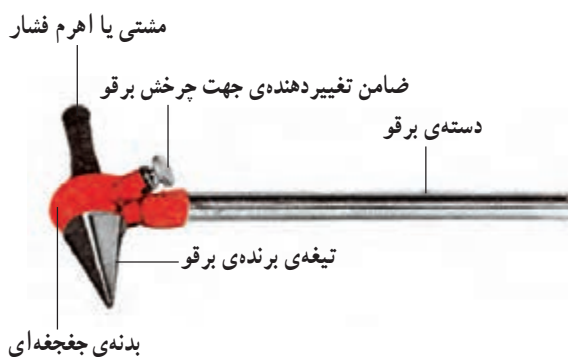
شکل ۹-۲- اجزای برقی جفجغه‌ای
