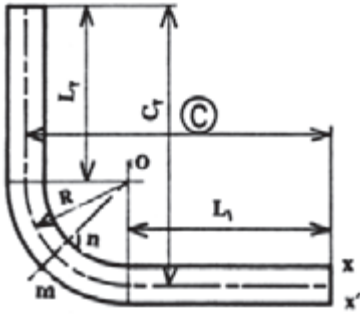
شکل ۳۲-۳- قطعه‌ی خم کاری شده
