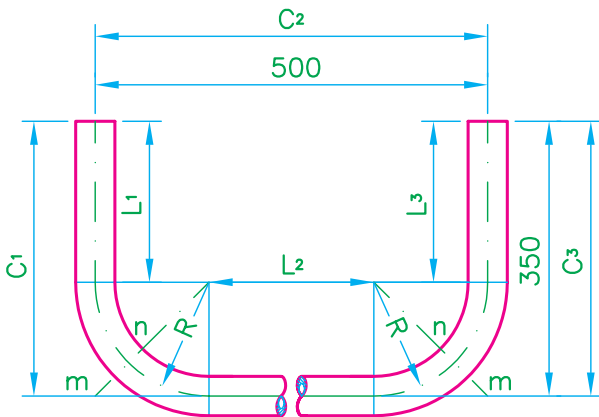
شکل ۳۴-۳- کلاف زیر دست شویی بدون پایه‌ی ۵۲ سانتی متری
