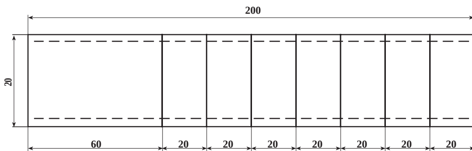
نقشه‌ی کار (۳)
