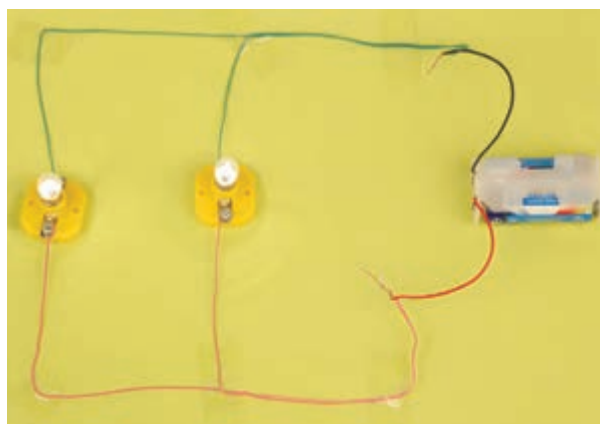
مدار موازی
