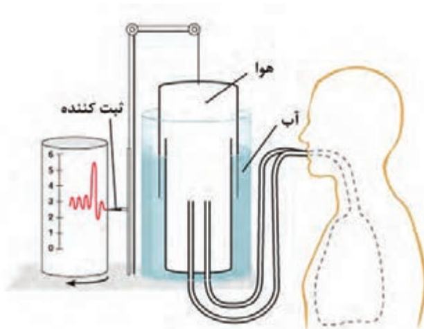
ساختار کلی یک اسپرومتر استاندارد
