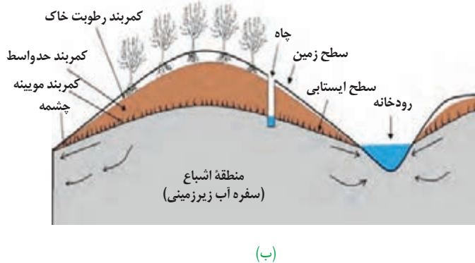
شکل ۳-۳ الف) توزیع آب زیرزمینی در خاک، ب) کمرندهای منطقه تهویه
