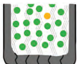
شکل ۲۴- سوختن گاز هیدروژن
