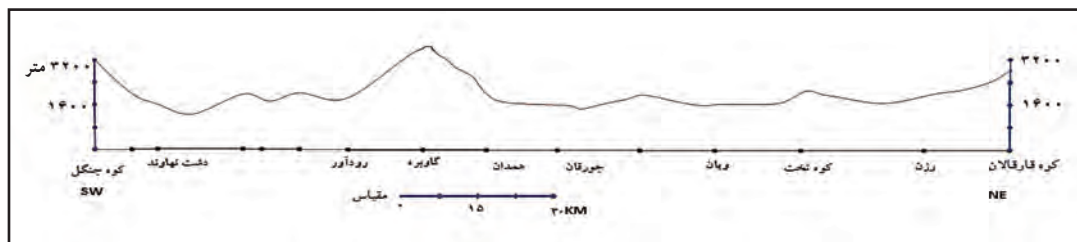
شکل ۳-۱. نیمرخ ناهماری های استان در جهت جنوب غرب - شمال شرق (از ناهاند تا رزن)
