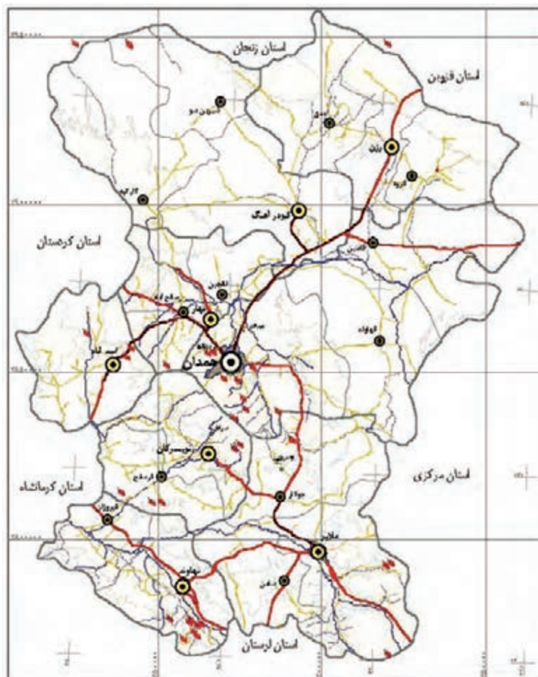
شکل ۱۴-۱ نقشه محدوده فعالیت رانش زمین
