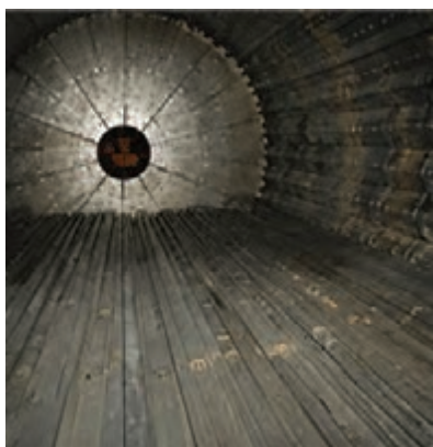
شکل ۱۸- نمای داخلی آسیاب میله‌ای
