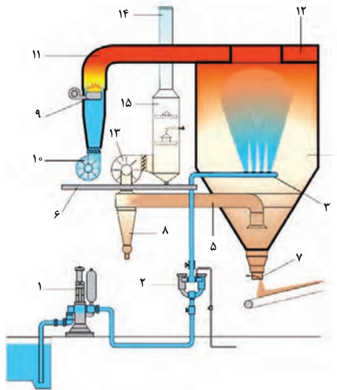
شکل ۱۵- نمایی از اجزای خشک کن پاششی
