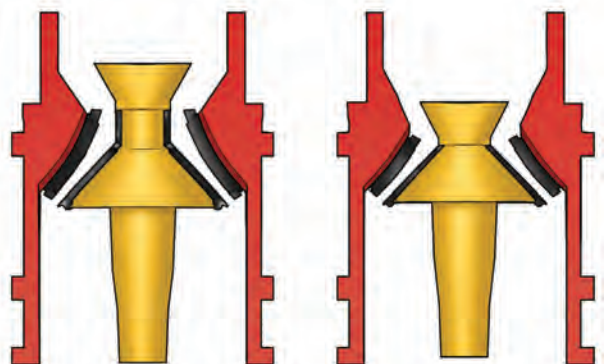
الف) کلاhek کوتاه ب) کلاhek بلند شکل ۳۲- انواع سنگ‌شکن مخروطی
