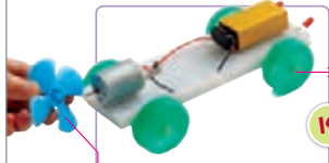
۱۴ پروانه را وصل کنید. حالا وقتی کلید را دوباره می‌زنید، خودروی شما آماده حرکت است. اگر چرخیدن پروانه، خودرو رو به جلو حرکت نمی‌کند، سیم‌های موتور را طوری تغییر دهید که محور موتور برعکس حالت قبیل بچرخد.
