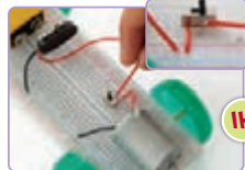
۱۳ اتصال دهنده پایه‌های باتری را به آن وصل کنید. با استفاده از سیم چین حدود نیم سانتی‌متر از روکش هر دو انتهای سیم‌های اتصال دهنده را بردارید.
