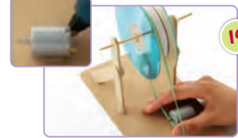
۱۹ موتور را بین دو ستون و در مکانی مناسب به گونه‌ای یا چسب حرارتی به تخته لکچیان بچسبانیید تا وقتی کش لاستیکی را روی محور موتور قرار می‌دهید، به قدر کافی محکم باشد.
