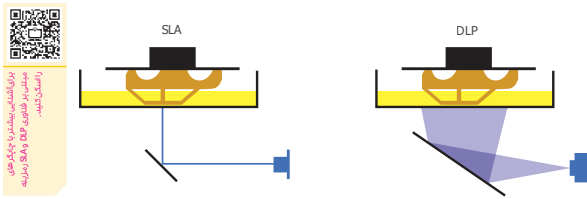
شکل ۷ مقایسه تابش به رزین در فناوری SLA و DLP
