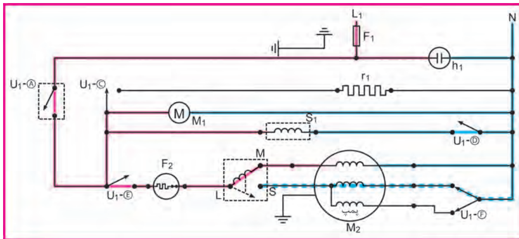
ت - نقشه تفکیکی سیم بندی ظرفشویی اتوماتیک با الکتروپمپ دو جهته در مقطع زمانی بین ۹ و ۱۰
