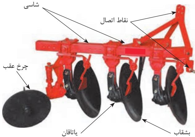
شکل ۸-۱. گاوآهن بشقابی
