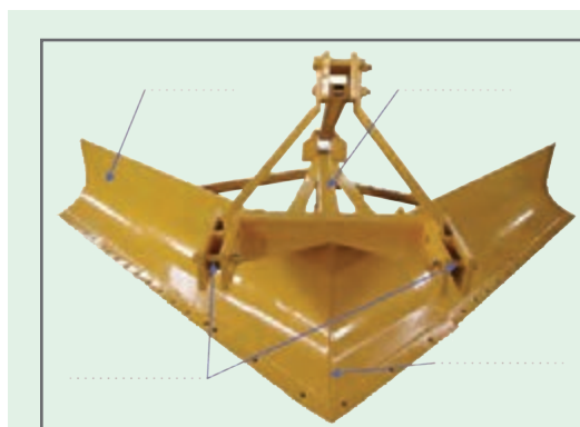
شکل ۲۱- ساختمان نهرکن
