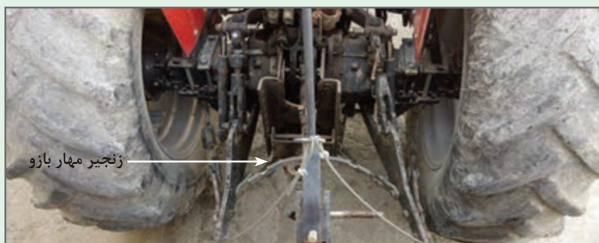
شکل ۱۴- زنجیر مهار بازوی تراکتور
