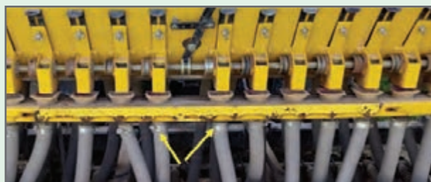
شکل ۲۸- بست‌های نگهدارنده لوله‌های سقوط
