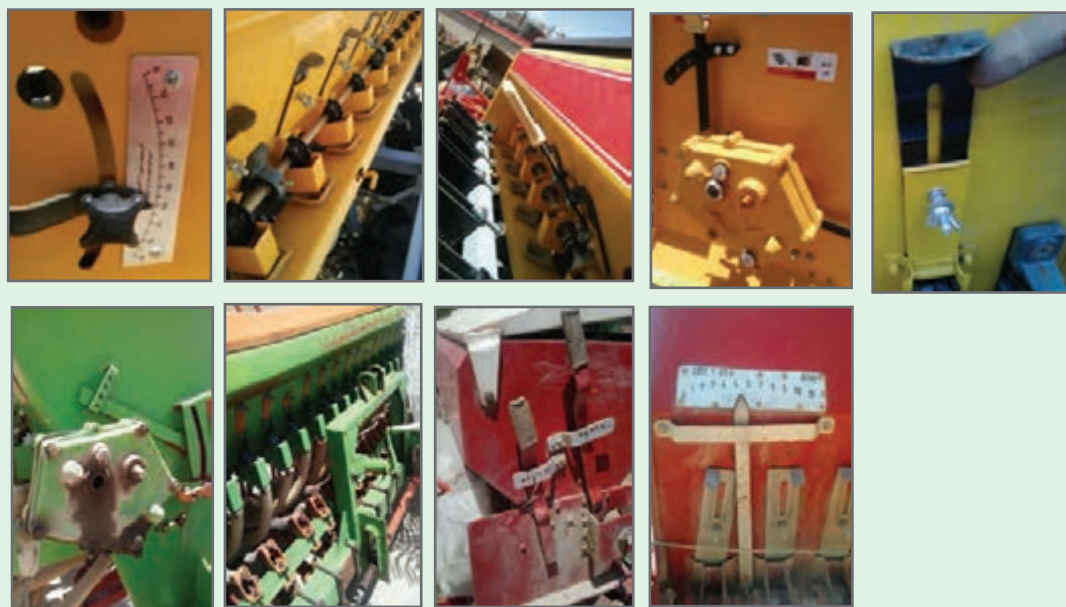
شکل ۵۷- برخی از تجهیزات و ساز و کارهای تنظیم در انواعی از ماشین‌های کاشت دیم
