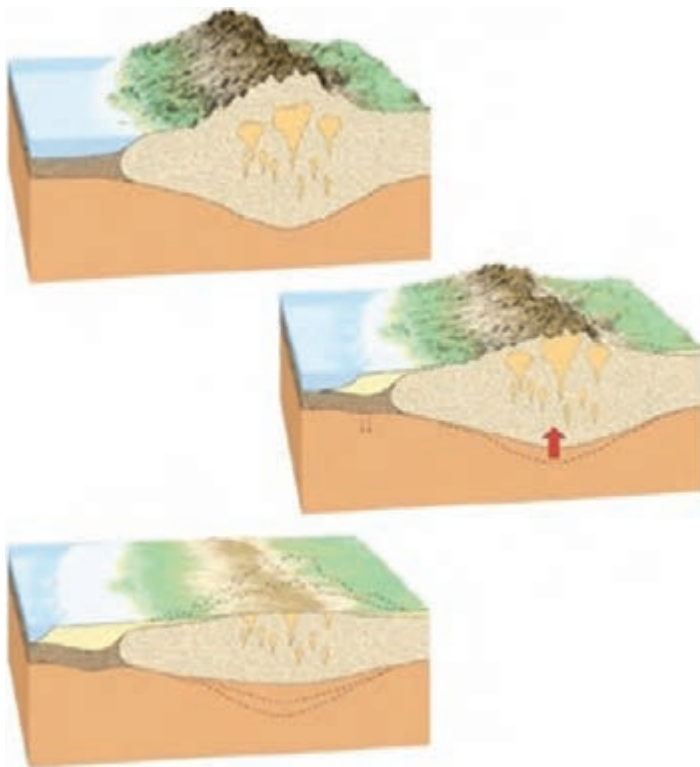
شکل ۲-۸- براساس اصل ایزوستازی پوسته جامد زمین در زیر قاره‌ها و اقیانوس‌ها همواره در حال تعادل است
