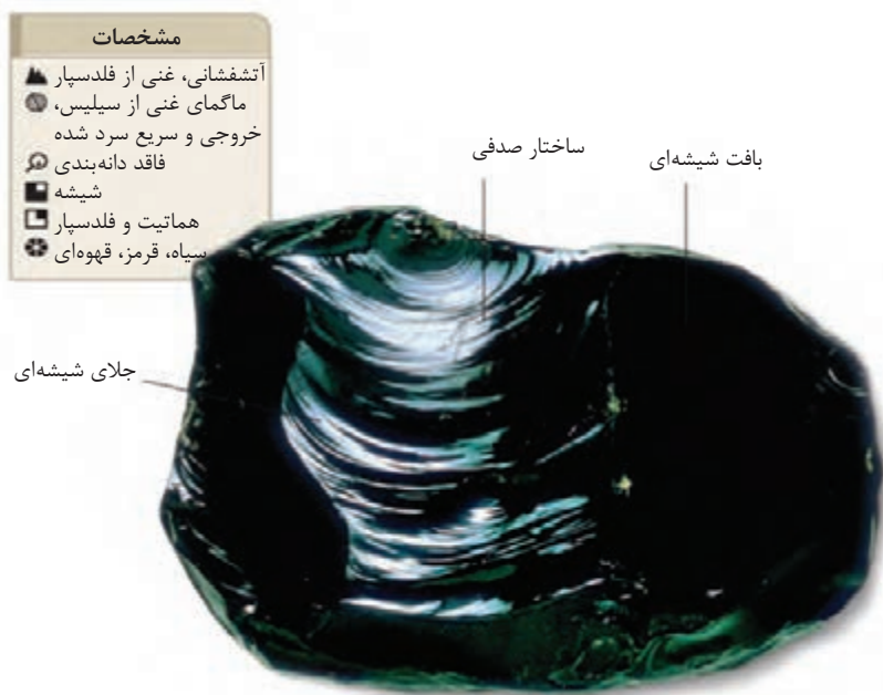
شکل ۲-۲۶- ابسیدین
