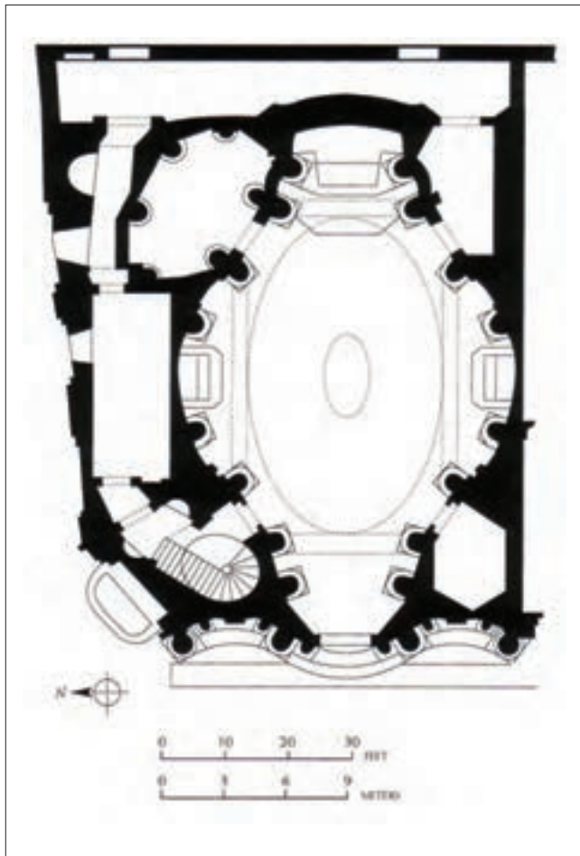
۵-۴ ب: نقشه کلیسای سان کارلو آله کوآترو فونتانه رم، برومینی
