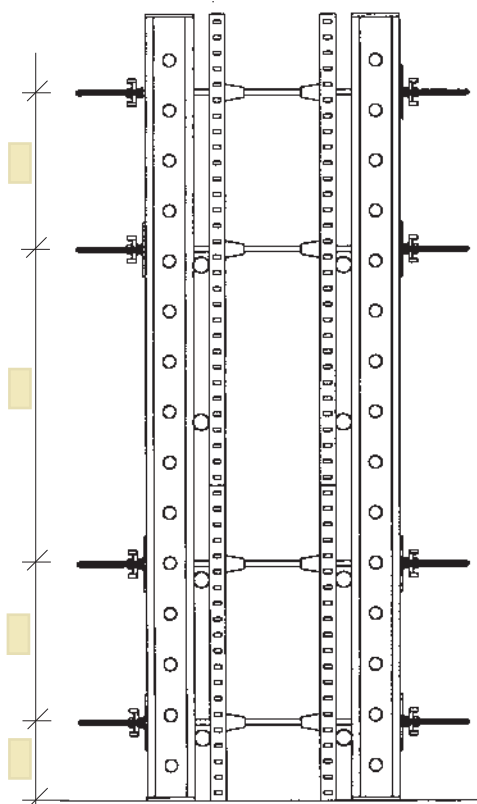
برش .....
