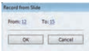
شکل ۱۱-۱۱- انتخاب اسلایدها
