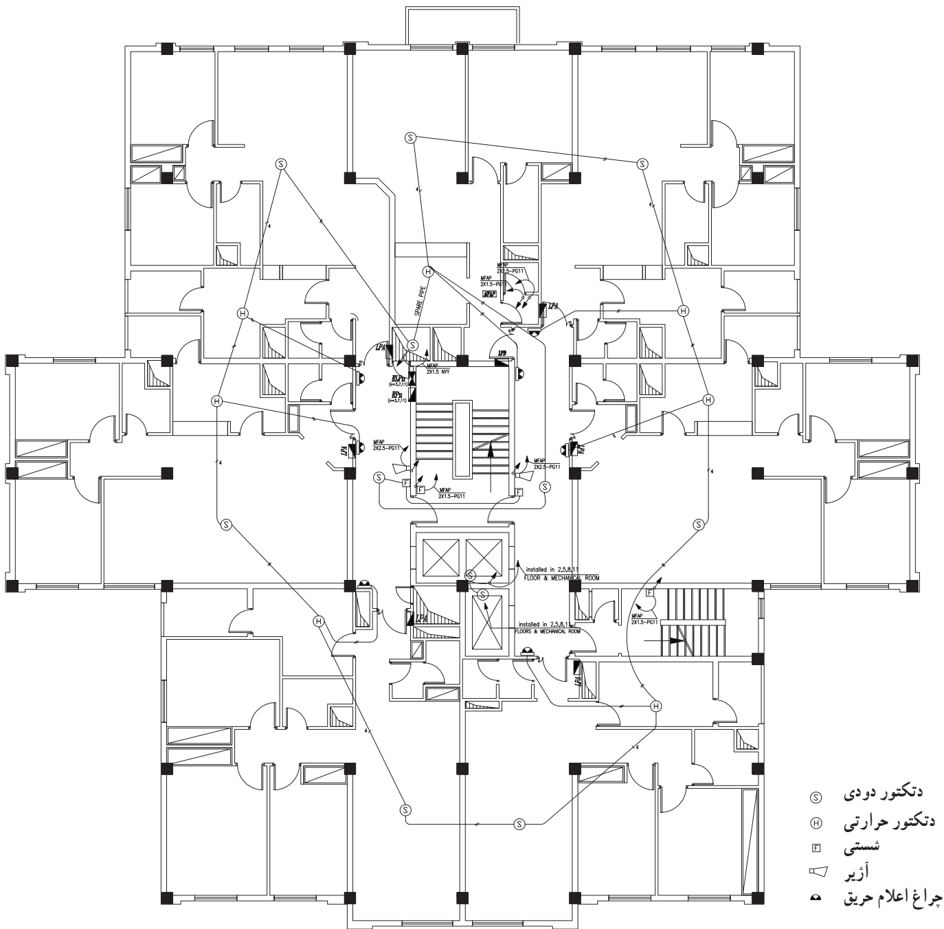
شکل ۱۲-۶ سیستم اعلام حریق یک طبقه با ۷ واحد مسکونی
