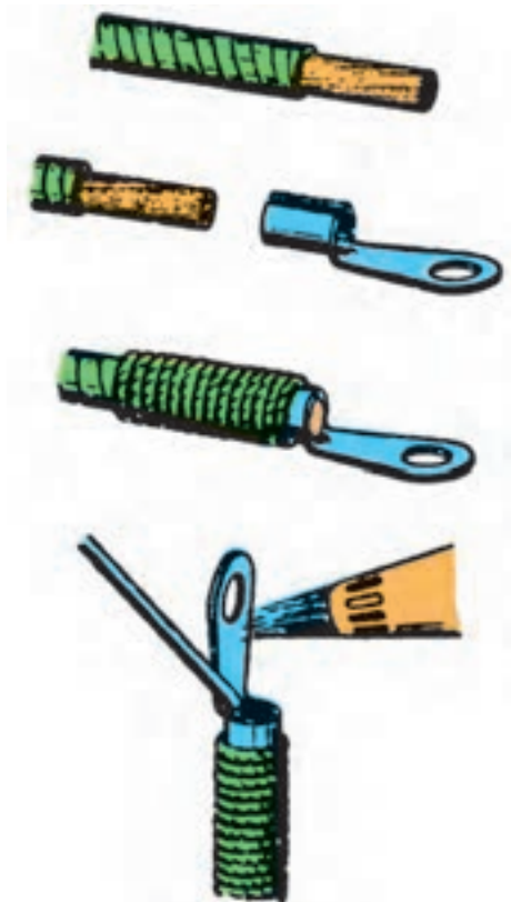
شکل ۲۸-۵- مراحل لحیم کاری کابل شو
