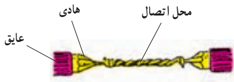
شکل ۱-۱-۱ نمونه‌ی اتصال دو سیم به یکدیگر
