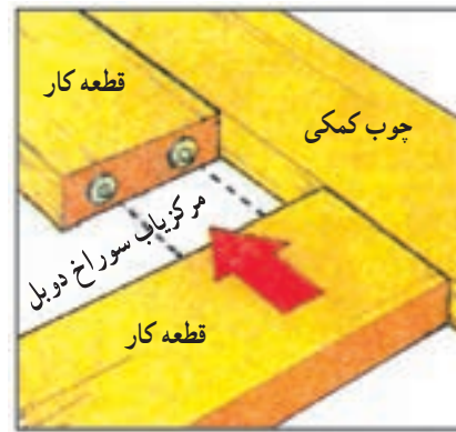
شکل ۱۰-۸- قطعه مرکز یاب سوراخ قطعه مجاور
