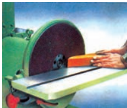
شکل ۸-۱۲- نحوه سنباده زدن قوس‌های محدب
