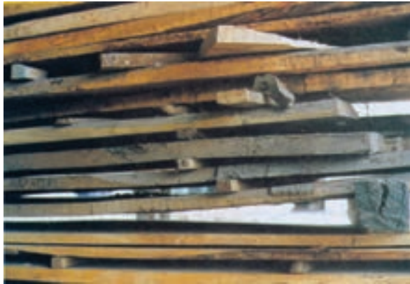
شکل ۱۳-۲- وجود یک چوبدستک ضخیم تر به کج شدن تخته ها می انجامد.
