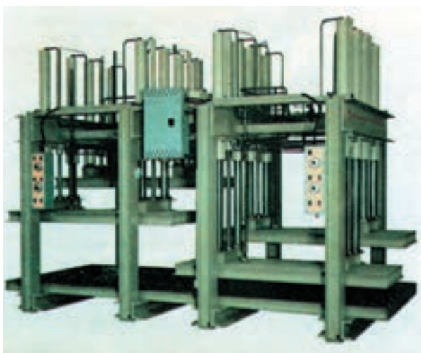
پرس سه قطعه‌ای با پیچ و فلکه جهت چسباندن روکشهای چوبی
