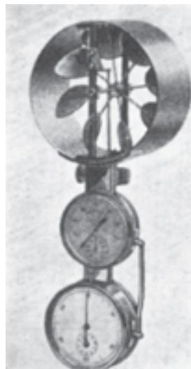
شکل ۲-۱-۸- هواسنج (آنومتر)
