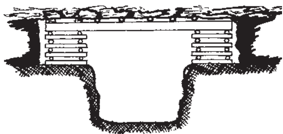
شکل ۵۸-۲۴- استفاده از جرزبندی به جای ستون
