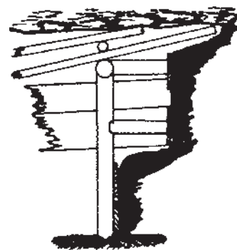
شکل ۱۳-۲۴- نحوه‌ی چیدن پاس در محیط‌های ریزشی
