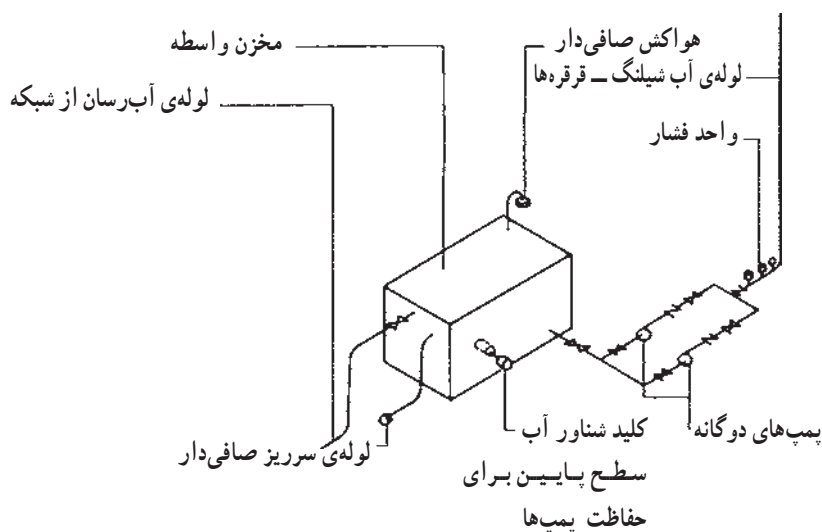
شکل ۱۲-۱۵- پمپ آتش‌نشانی
