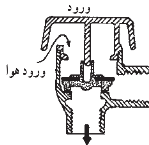
شکل ۵-۵ شیر خلاشکن شیر در حالت برگشت جریان عمل کرده است.
