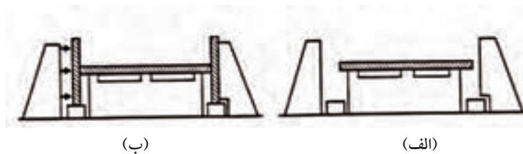
شکل ۱۱-۶- مونتاز تیرورق در قالب
