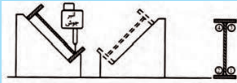
شکل ۱۱-۱۰- ترتیب و توالی و طرمراره اجرای جوش طولی تیر یا ستون در حالت تفت
