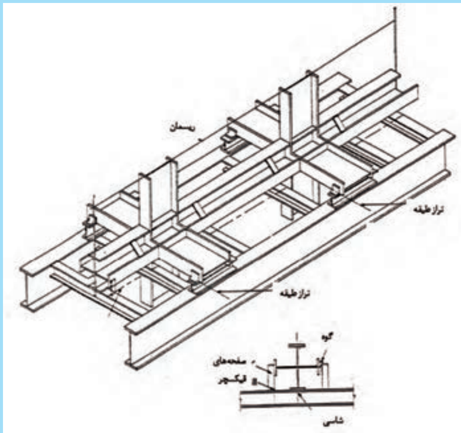
شکل ۱۱-۱۵- فیکسچر مونتاژ نهایی قطعات الماکی دستک‌ها روی ستون صلیبی شکل
