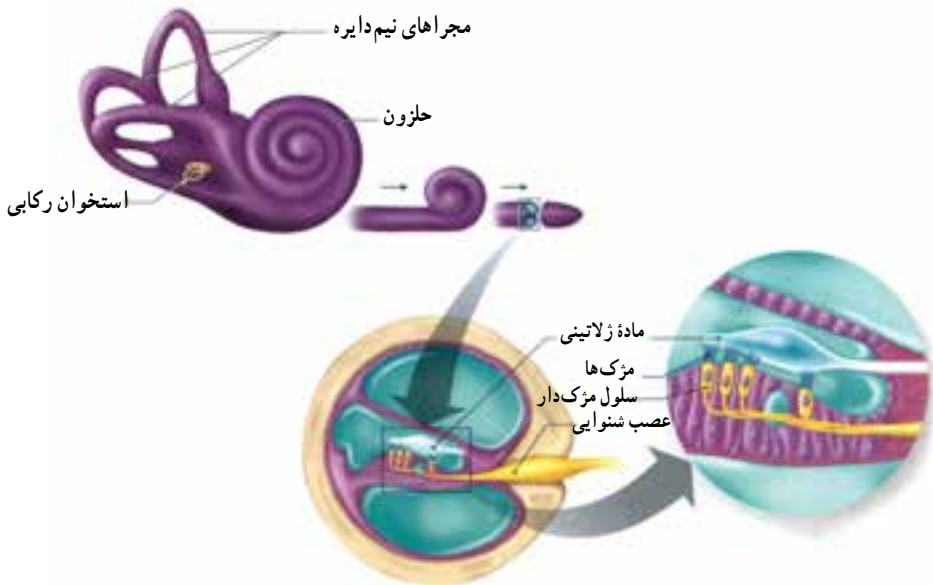
شکل ۷-۳- حلزون گوش
